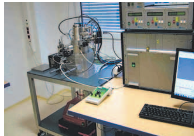
Низковольтная электронно-зондовая система для мониторинга дефектов
